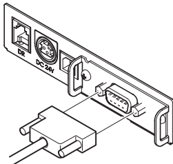
Serial RS-232C cable
