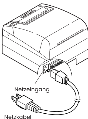
Ausführung mit Netzteil (integriertes Netzteil)
