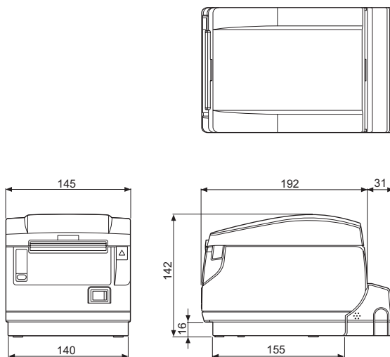
Tipo con fuente de alimentación integrada
