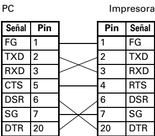
Cable de 25 pines – 25 pines
