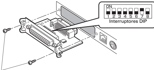
Tornillos de fijación de la tornillos de fijación de la placa de interfaz serie
